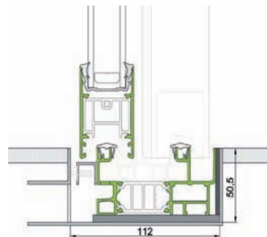
Kolejničky zapuštěná PMR. 2-kolejničové posuvné řešení se zapuštěným spodním rámem s nerezovou vaničkou
