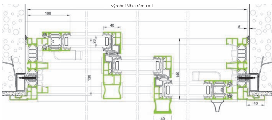
řez provedení 3 kolejničky
