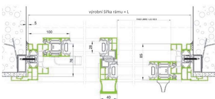
řez provedení 2 kolejničky
